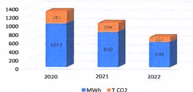
Energía térmica (MWh) Y CO2 (T)
